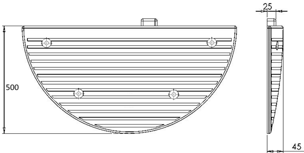
K901 – Capac limitator de viteza:
