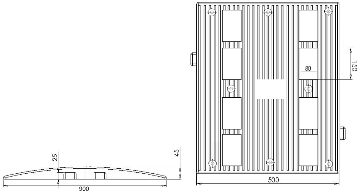
K901 – Capac limitator de viteza:
